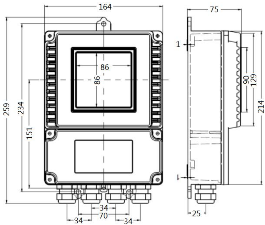
图 6c 211E 壳体分体式尺寸图
