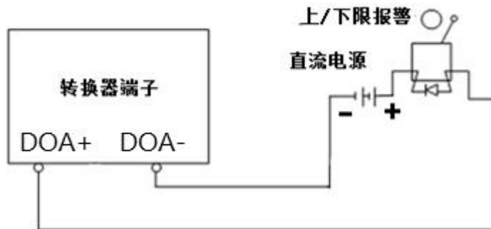
图 1.3.3 报警输出接线
