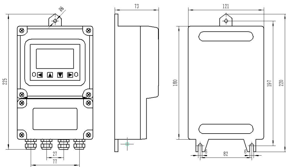
图 6d 211S 壳体分体式尺寸图
