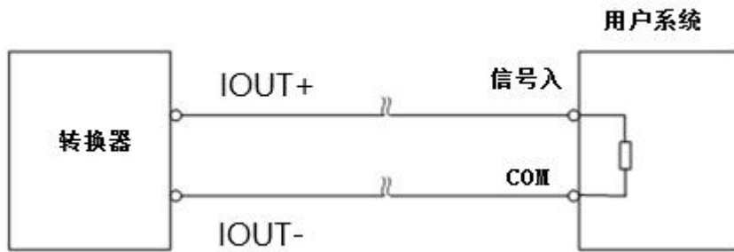
图 1.3.1 4~20mA 内供电接法
