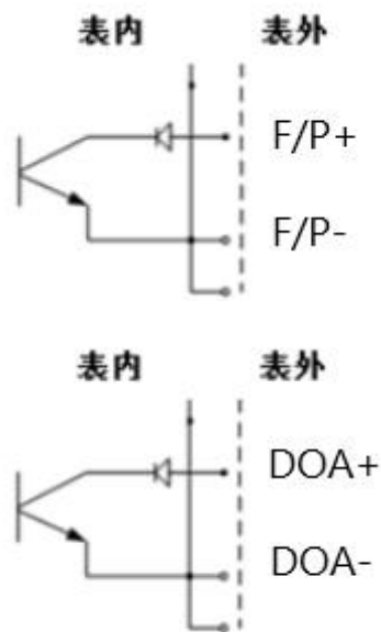
图 1.3.4 表内 OC 门连接方式
