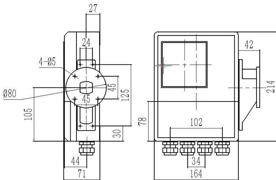
图 6a 211B 壳体一体式尺寸图
