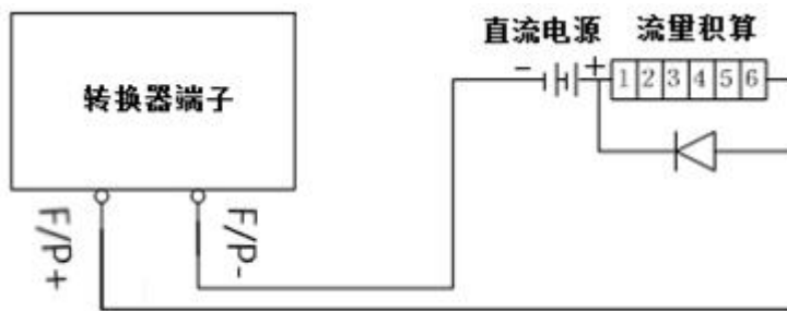
图 1.3.2 外供电接电子计数器
