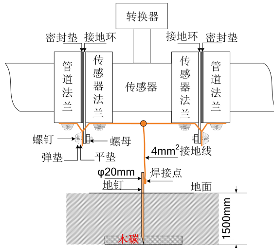
图 1.2.3 转换器接地示意图
