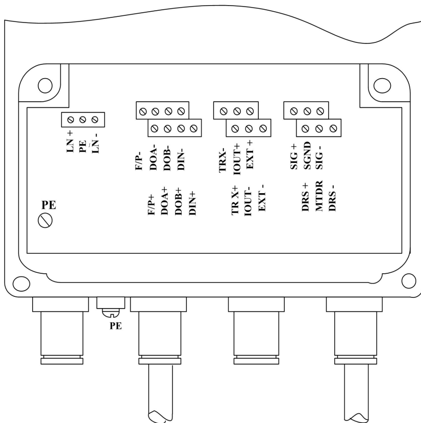
图 1.1.1 方表接线端子图
