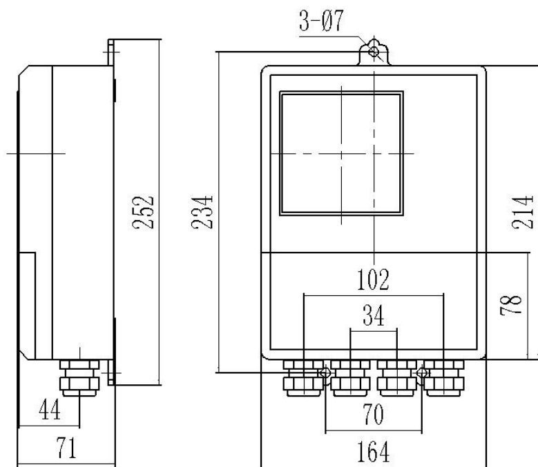
图 6b 211B 壳体分体式尺寸图
